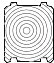
HH 142x160
