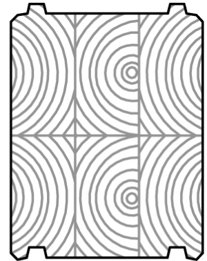
LHV 205x260
