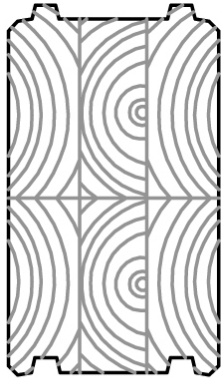
LHV 155x260
