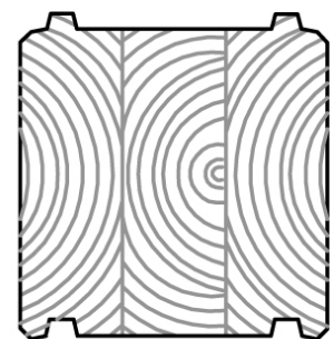
LH 205x205
