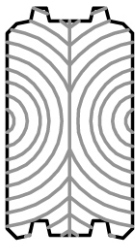
LH 95x160
