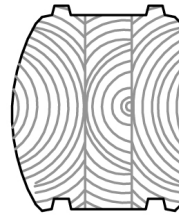
DLH 180x205
