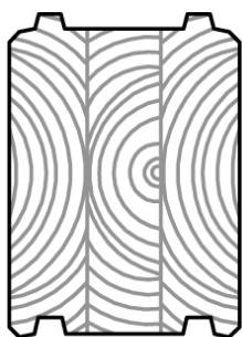
LH 155x205
