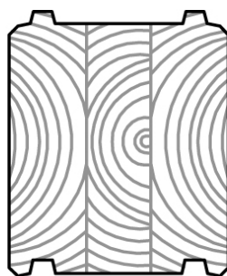
LH 180x205
